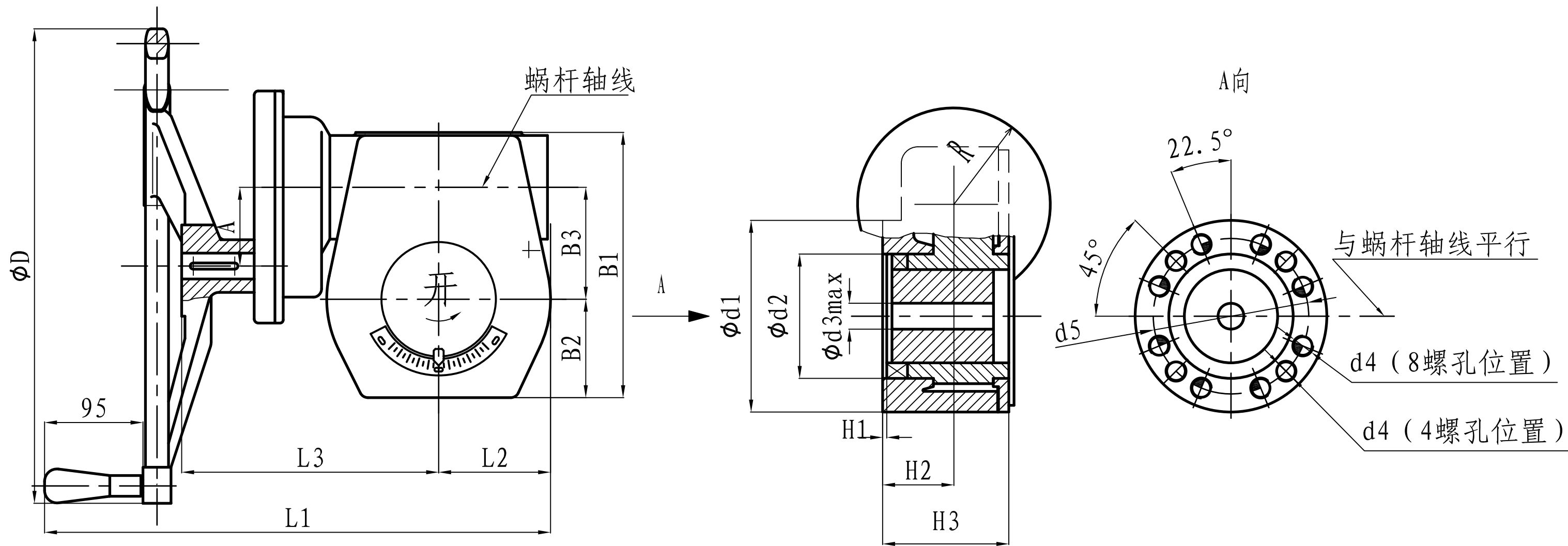
VGC-20、35、70外形及连接尺寸
